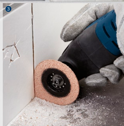
3 Režkanje fug tudi v kotu 90 stopinj.
