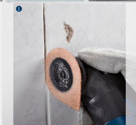
1 Režkanje fug med stenskimi in talnimi ploščicami.
